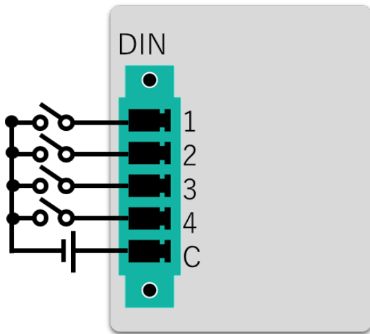
デジタル出力接続例
