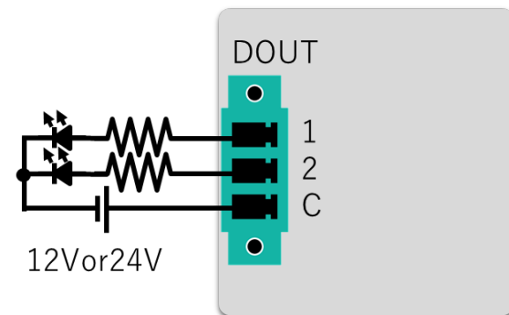
LED 接続例
